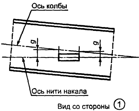
Рисунок 7 — Эксцентриситет оси колбы 10)
