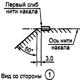
Рисунок 4 — Зона без металлических частей 8)
