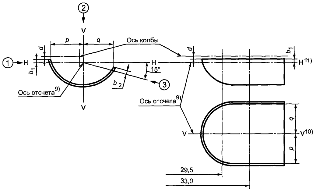
Расположение экранирующей части колбы*)
