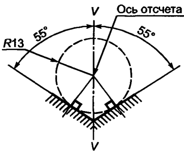
Рисунок 3 — Определение оси отсчета 2)
