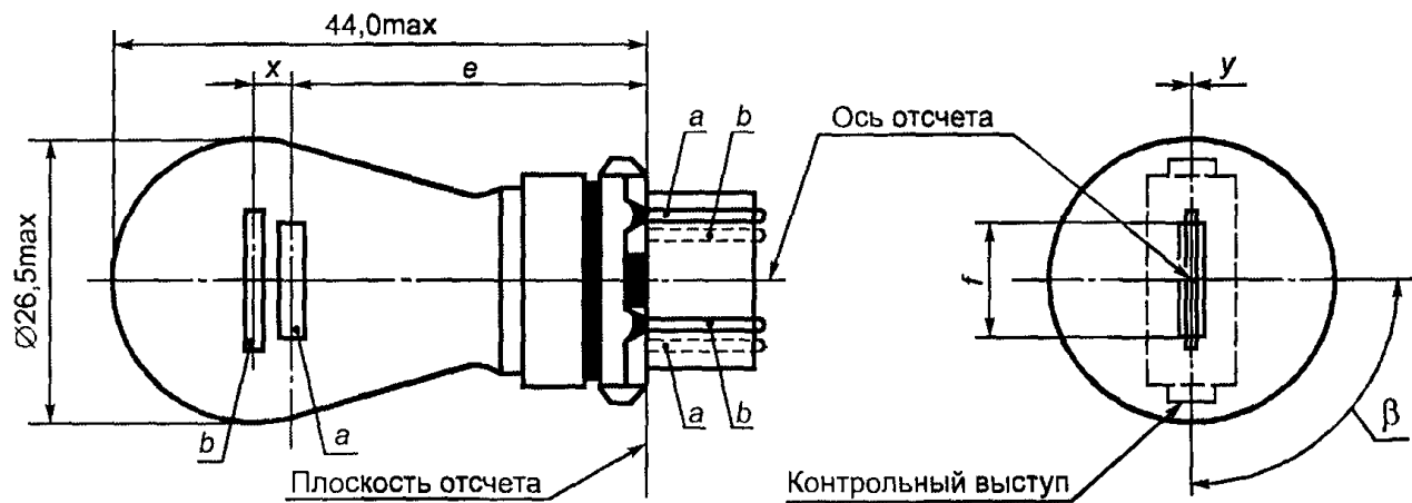
a — основная (с высокой номинальной мощностью) нить накала; b — вспомогательная (с низкой номинальной мощностью) нить накала
