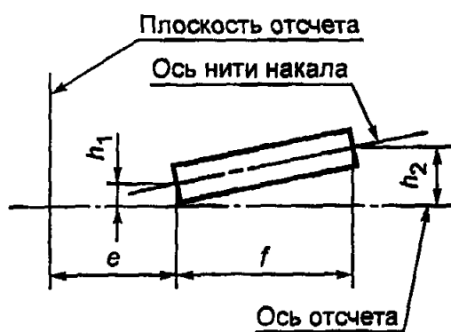
Рисунок 5 — Смещение нити накала 7) (только для эталонных ламп накаливания)
