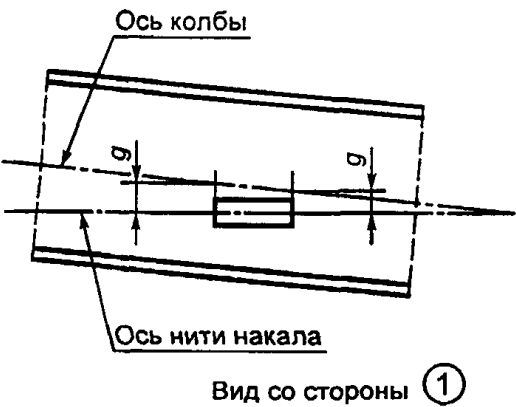
Рисунок 6 — Эксцентриситет оси колбы 10)
