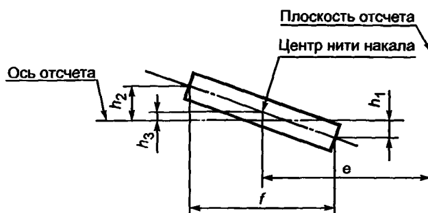
Положение нити накала и размеры
