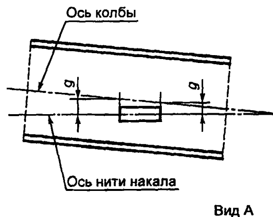
Рисунок 6 — Эксцентриситет оси колбы 8)
