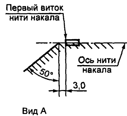
Рисунок 4 — Зона без металлических частей 6)
