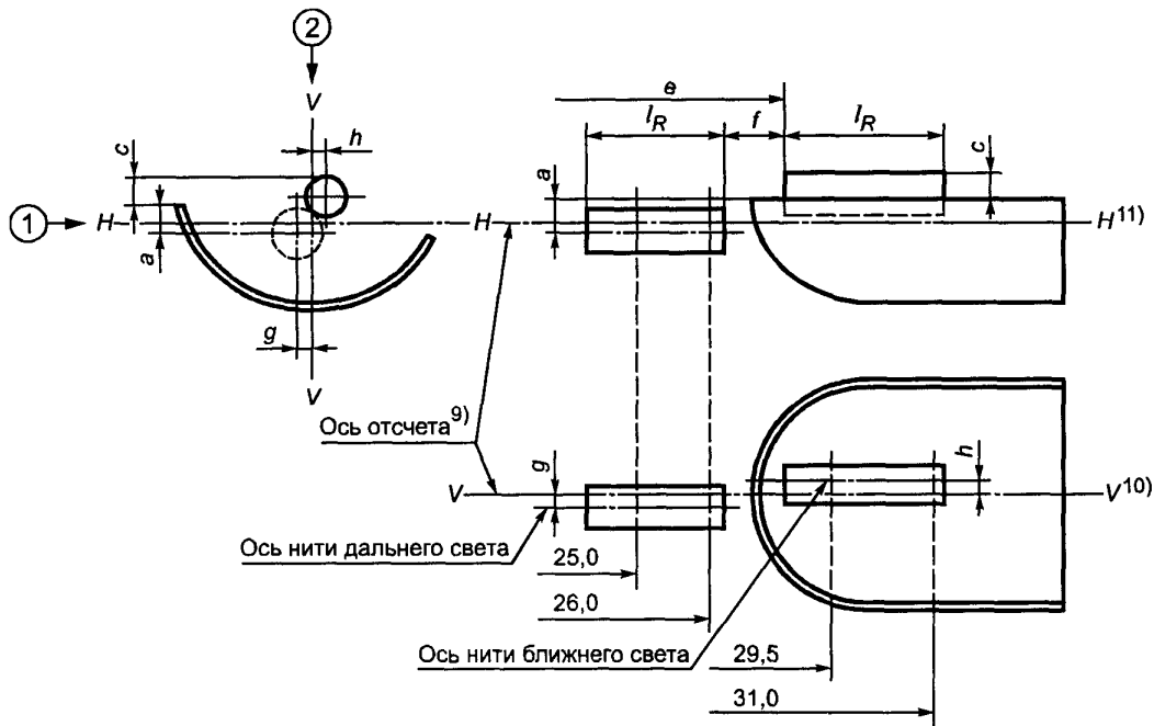
Расположение нитей накала*)
