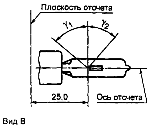
Рисунок 3 — Зона без оптического искажения 5)
