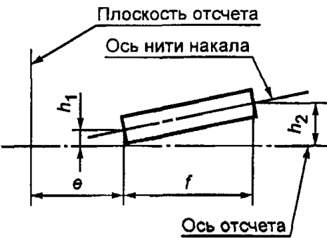
Рисунок 5 — Допустимое смещение оси нити накала 9) (только для эталонных ламп накаливания)
