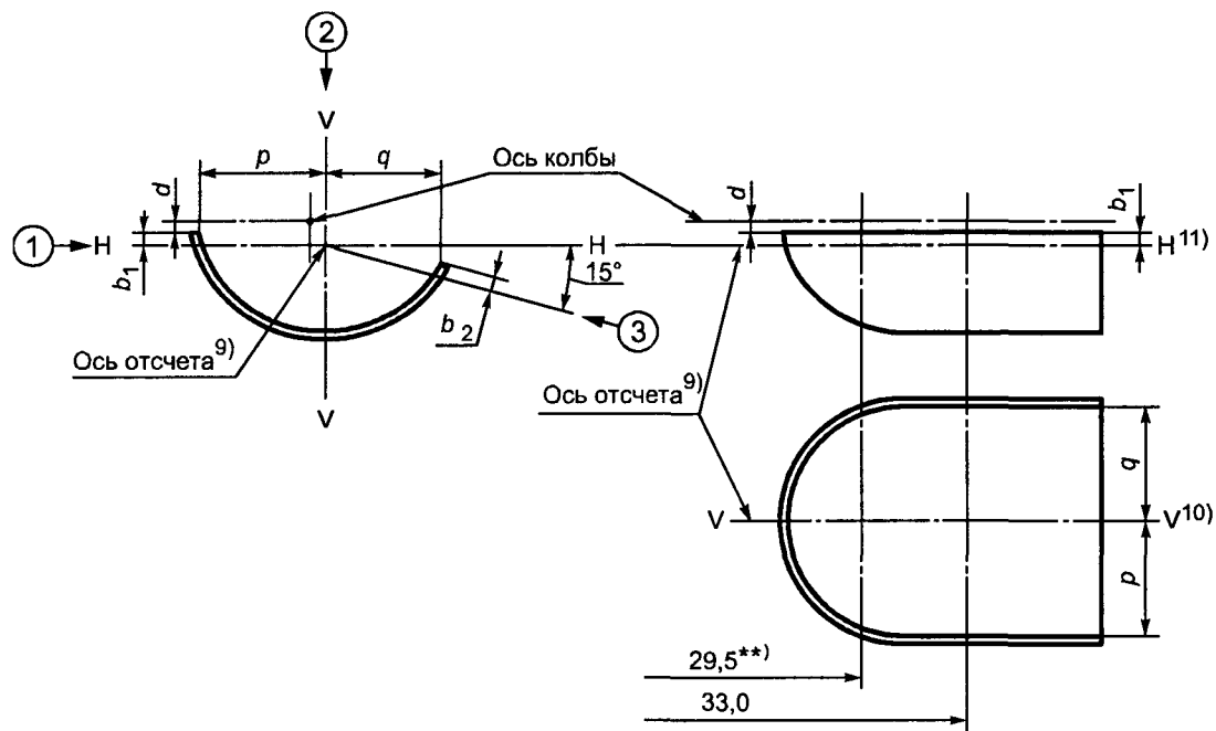
Расположение экранизирующей части колбы*
