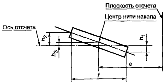
Положение нити накала и размеры
