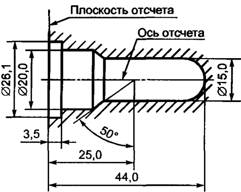
Рисунок 2 — Максимальные размеры лампы 3)
