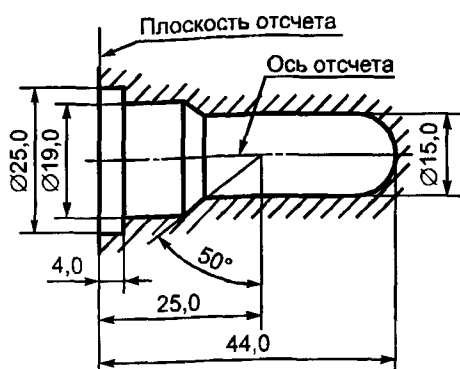
Рисунок 2 — Максимальный внешний контур лампы 3)
