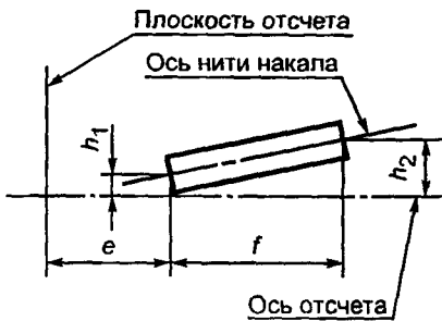
Рисунок 6 — Допустимое смещение оси нити накала (только для эталонных ламп накаливания) 9)
