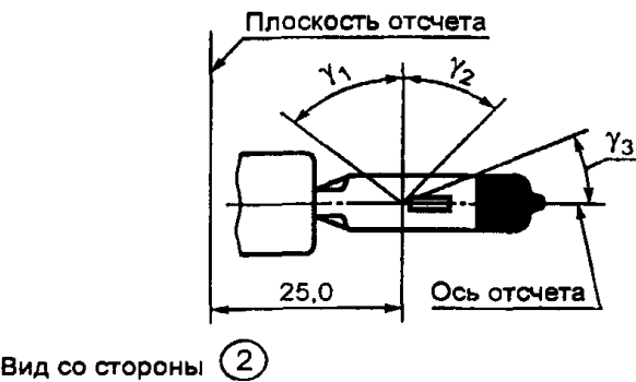
Рисунок 3 — Зона отсутствия искажения 6) и черная верхняя часть 7)
