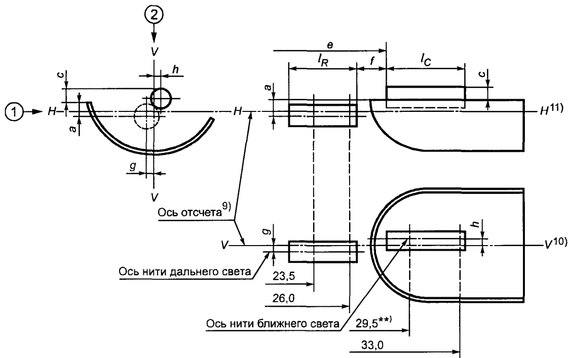
Расположение нитей накала*
