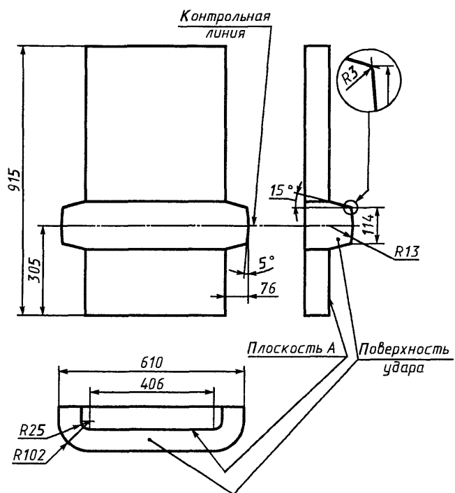
Рисунок 3.1 — Ударное устройство
