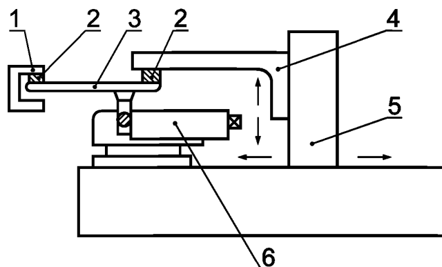
1 — нагрузка; 2 — металлические прокладки; 3 — защитный корпус; 4 — регулируемый упор; 5 — регулируемая опора; 6 — механизм блокировки
