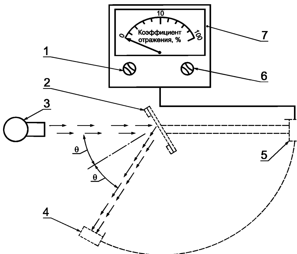
1 — установка на ноль; 2 — штатив для закрепления образца; 3 — источник света и коллиматор; 4 — приемное устройство с фотоэлементом в положении для измерения и «косвенного» градуирования; 5 — штанга приемного устройства в положении для прямого градуирования; 6 — регулировка градуирования; 7 — регулируемый индикатор
