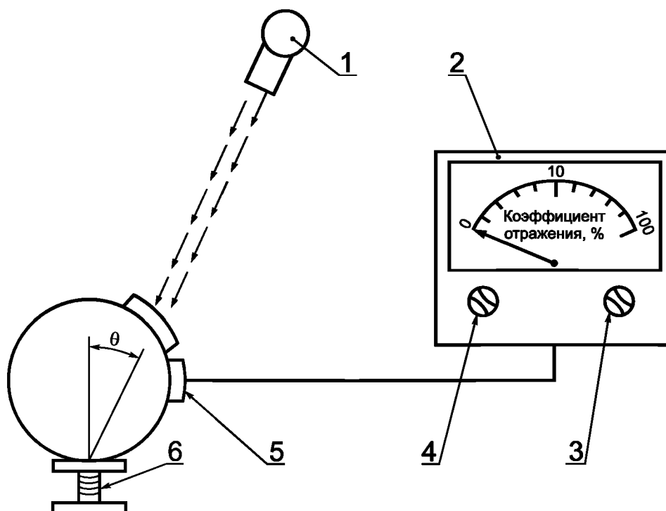
1 — источник света и коллиматор; 2 — регулируемый индикатор; 3 — регулировка градуирования; 4 — установка на ноль; 5 — фотоэлемент; 6 — штатив для закрепления образца
