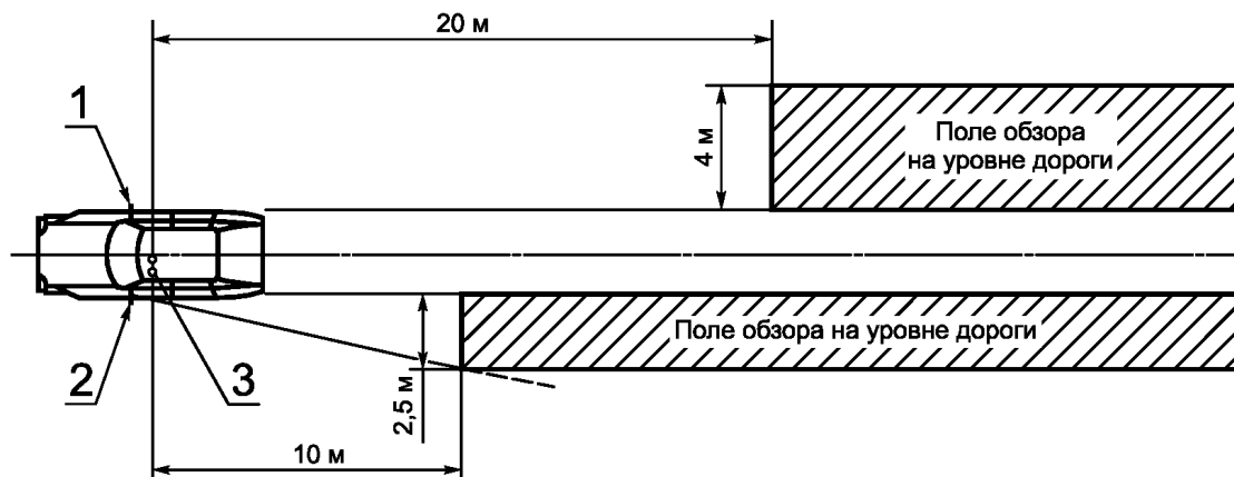
Рисунок 2 — Транспортные средства категорий M_1 и N_1 весом 2 т или менее
