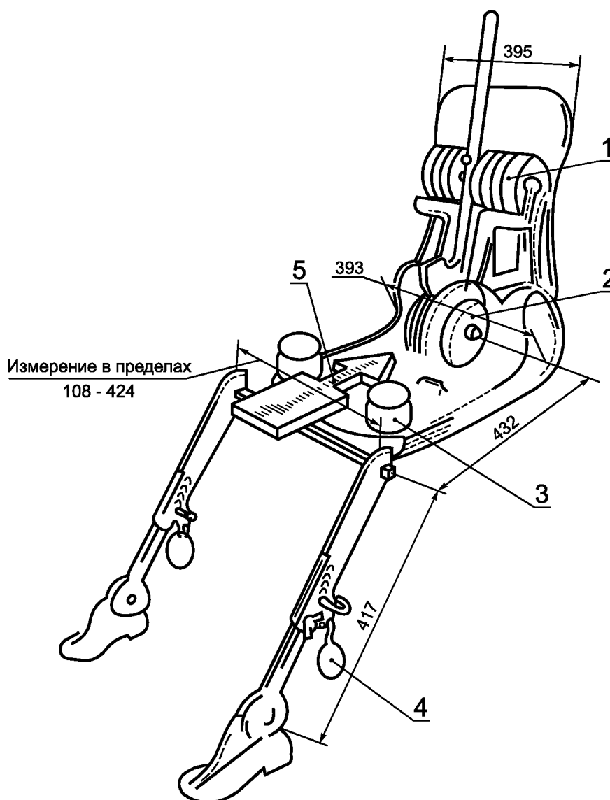
1 — спинные грузы; 2 — сидалишные грузы; 3 — набедренные грузы; 4 — ножные грузы; 5 — направление и точка приложения нагрузки
