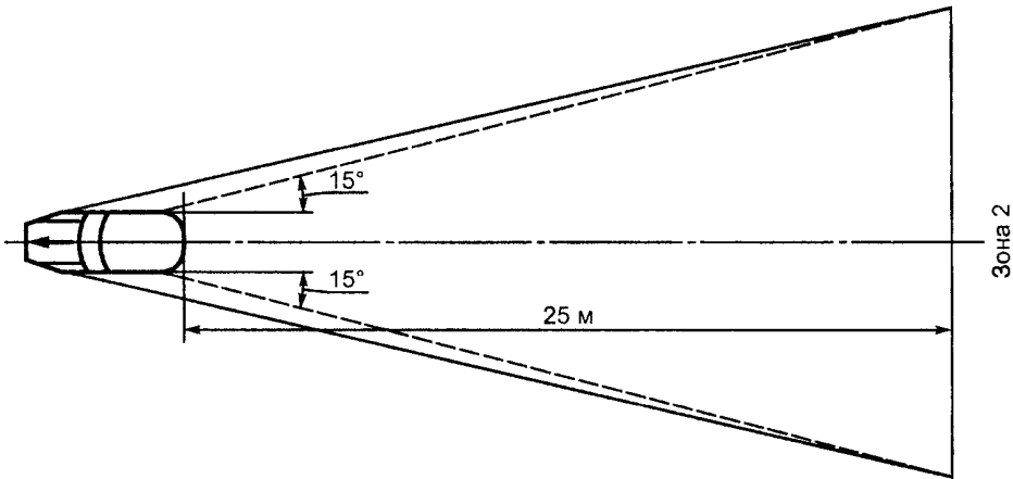
Рисунок 4.2 — Видимость белого огня в направлении назад
