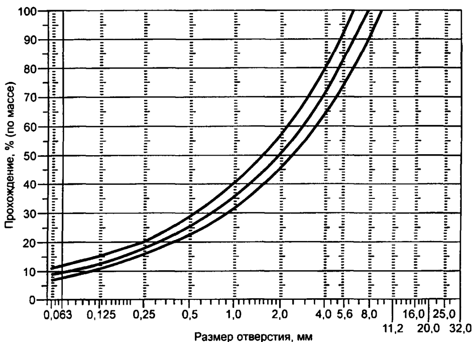
Рисунок 2 — Гранулометрическая кривая, отражающая состав скелетного материала асфальтобетонной смеси, с допусками
