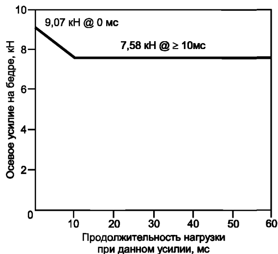
Рисунок 3 — Критерий нагрузки на бедра
