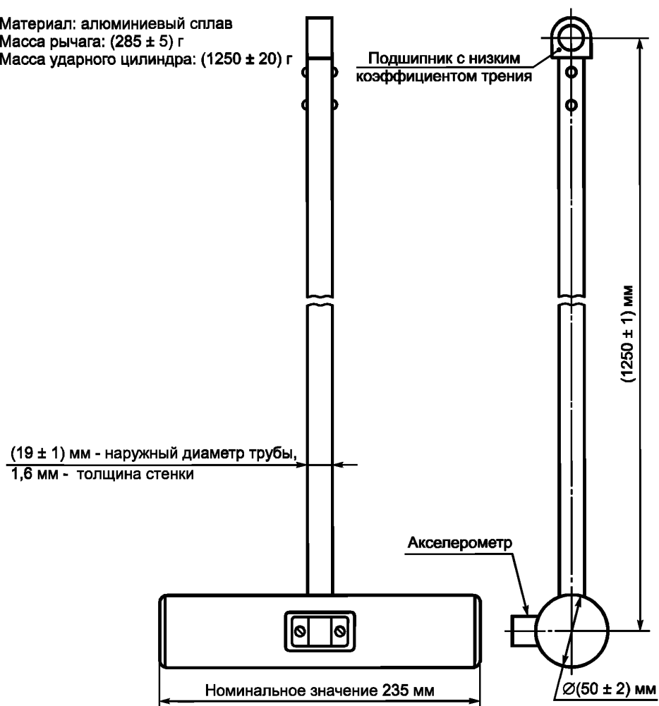
Рисунок 3а — Маятниковый ударный элемент
