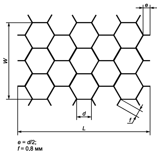
Рисунок 3 — Оси сотовой структуры и измеренные размеры
