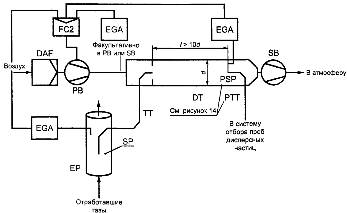
Рисунок 6 — Система разрежения части потока с измерением концентрации \text{CO}_2 или \text{NO}_x и частичным отбором проб
