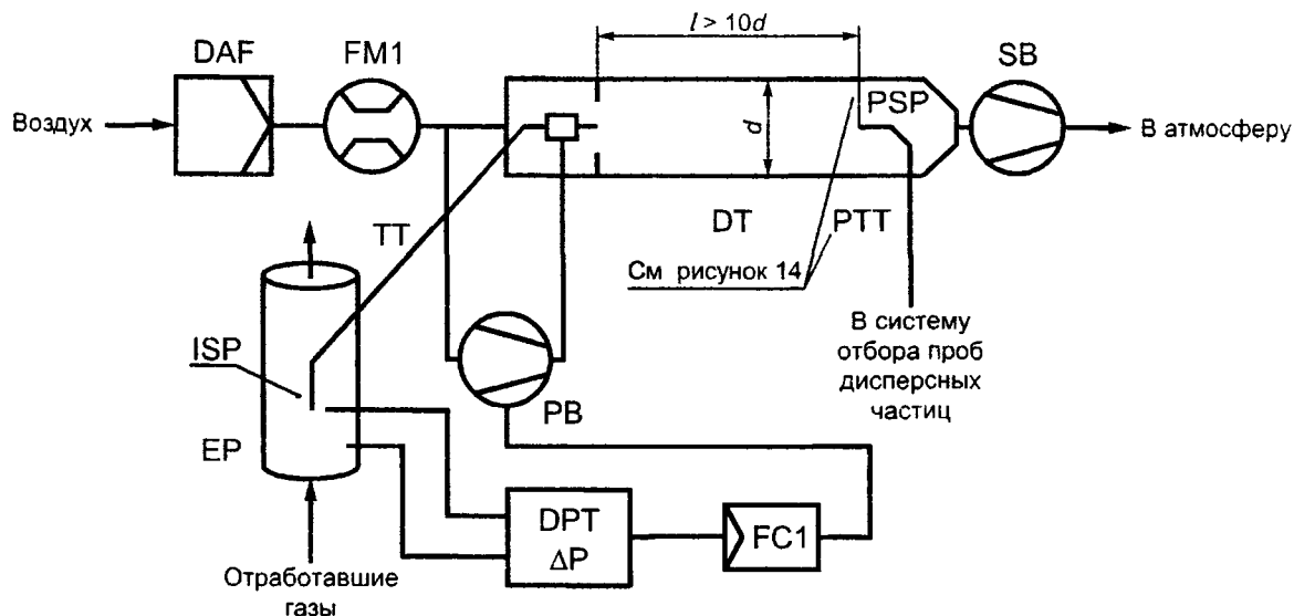
Рисунок 5 — Система разрежения части потока с изокINETическим пробоотборником и частичным отбором проб (контроль РВ)
