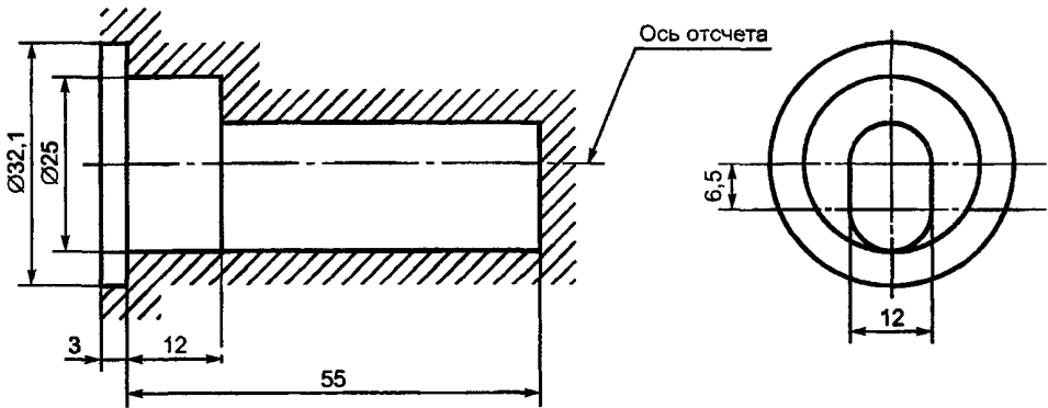
Рисунок 1.4 — Максимальный внешний контур лампы 2)
