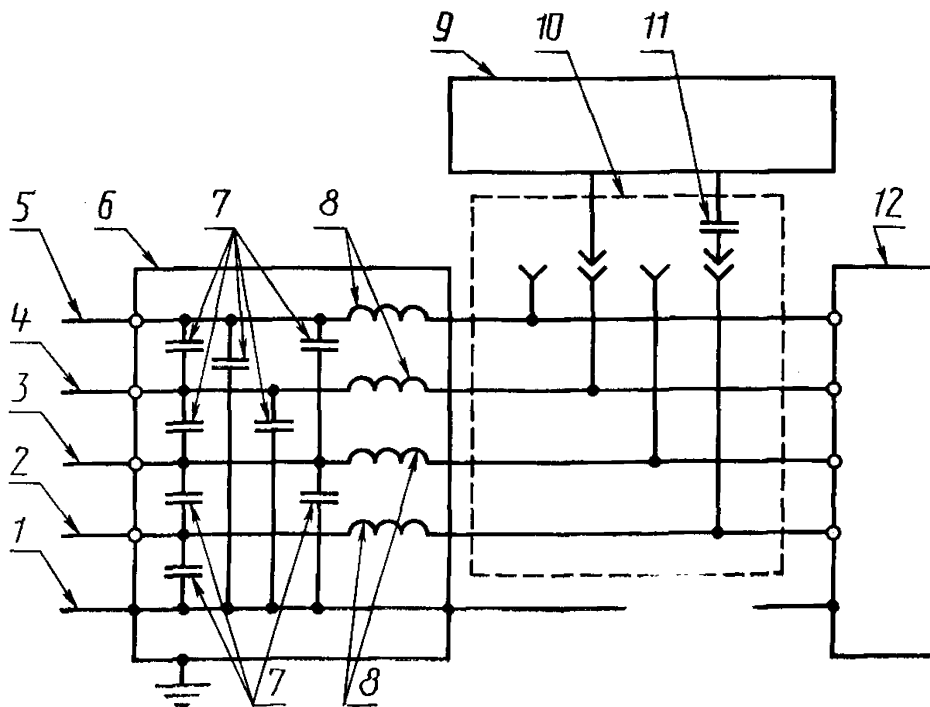
1, 2, 3, 4, 5 — защитный, нейтральный и фазные провода сети электропитания соответственно; 6 — устройство развязки; 7 — конденсаторы развязки; 8 — индуктивности развязки; 9 — ИГ МИП; 10 — устройство связи; 11 — конденсатор связи; 12 — ИТС
