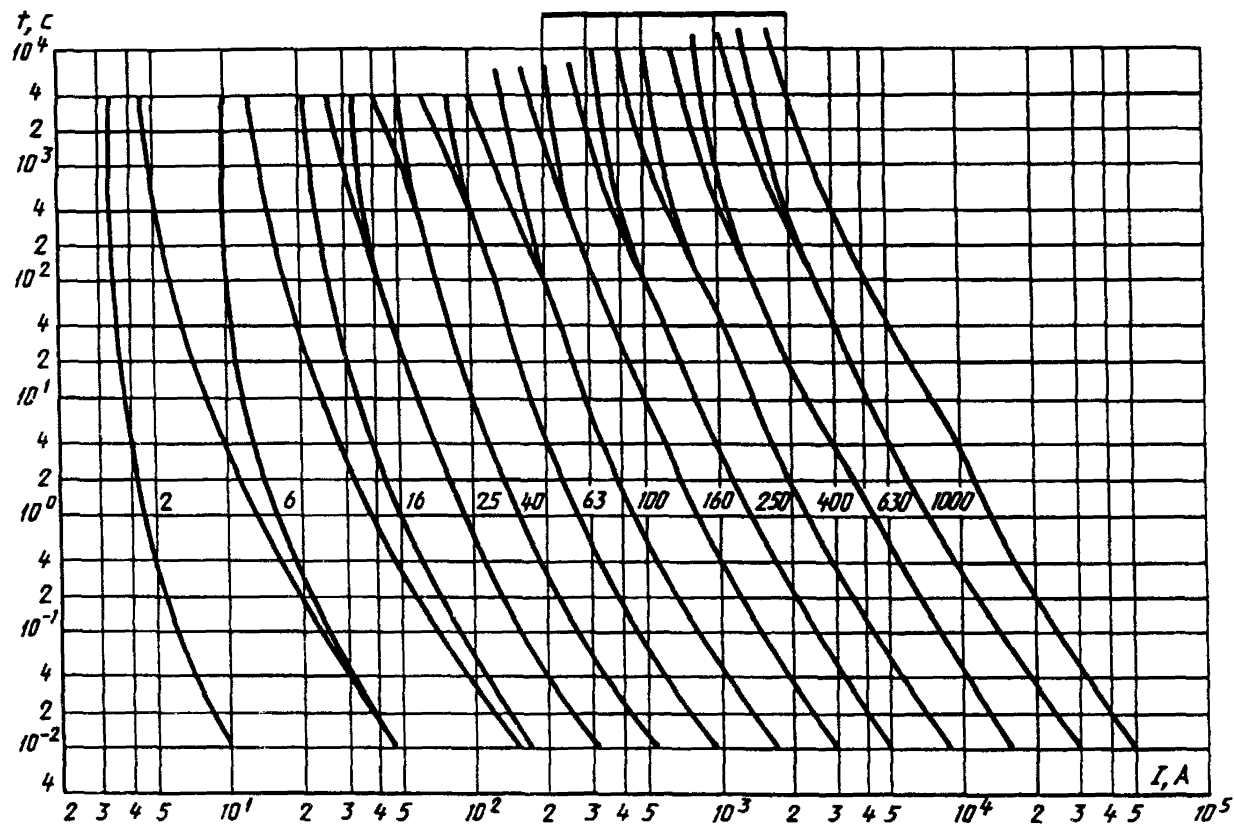
Черт. 4(П). Зона времятоковых характеристик плавких вставок gG
