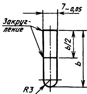
Черт 7 (I) Испытательный нож по п 8 5 5 1 2
