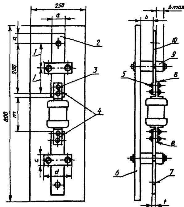
Черт. 5 (П). Устройство для испытаний на потери мощности
