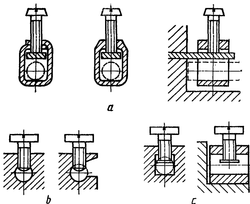
а) выводы с хомутиком; б) выводы без прижимных пластин; в) выводы с прижимными пластинами
