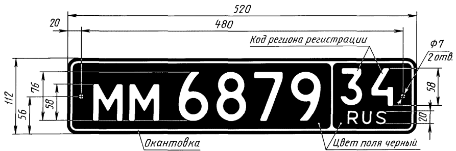
Рисунок А.9 — Регистрационный знак типа 6
