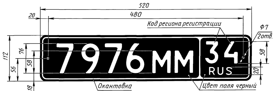
Рисунок А.8 — Регистрационный знак типа 5
