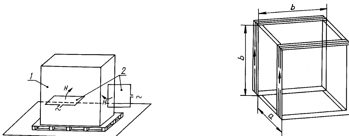
Рисунок 6 — Схема катушки Гельмгольца
