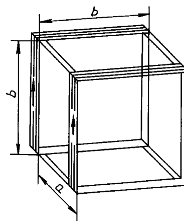
Рисунок 6 — Схема катушки Гельмгольца
