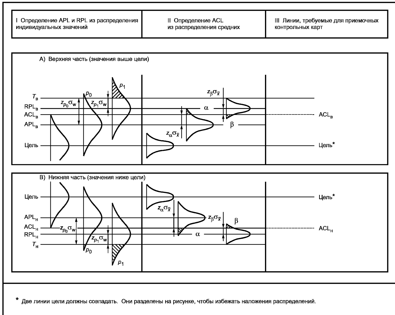
Рисунок 2 — Границы и определяющие элементы приемочных контрольных карт
