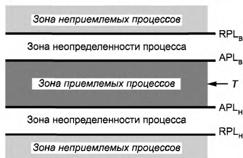
Рисунок 1 — Поле допуска: верхняя и нижняя линии APL и RPL в сопоставлении с зонами приемлемого, неприемлемого процессов и зоной неопределенности процесса
