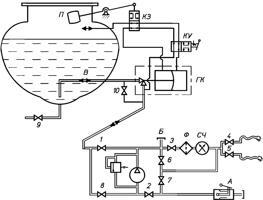
1—9 — задвижки; 10 — вентиль; А — напорно-всасывающий патрубок; Б — напорный патрубок; В — трубопровод для на- полнения и опорожнения; ГК — гидроклапан; П — поплавок; КЗ — клапан золотниковый; КУ — кран управления; Ф — фильтр; СЧ — счетчик
