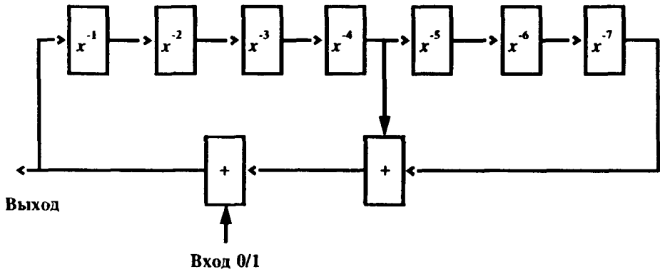
Рисунок 3 — Скремблер, реализующий полином 1 + x^4 + x^7
