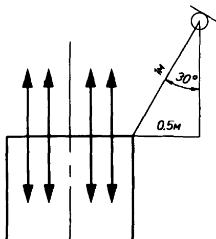
Рисунок А.2 — Измерительные точки у выпускной или всасывающей трубы
