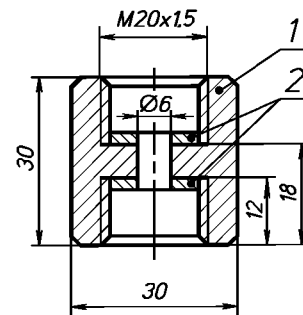
1 — переходник; 2 — прокладка
