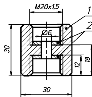
1 — переходник; 2 — прокладка
