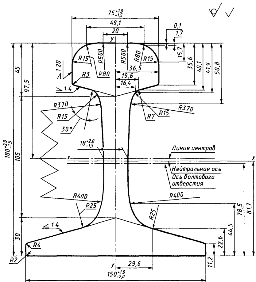
Рисунок 2 — Поперечное сечение рельса типа РР65
