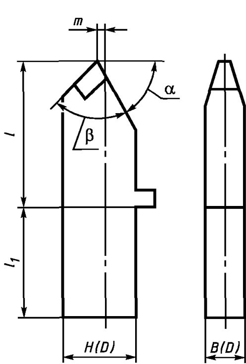
Рисунок 2 — Резец исполнения ТН
