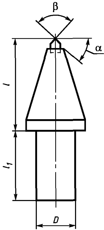
Рисунок 3 — Резец исполнения ТП
