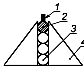
Размещение изделий по схеме № 2
