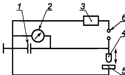
Рисунок 5 — Принципиальная схема установки для определения чувствительности ПИ к статическому электричеству
