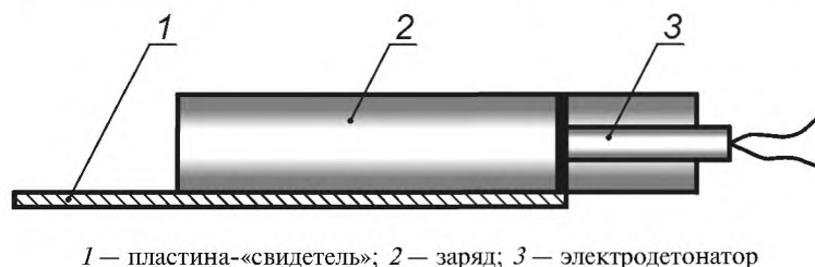
Рис. 3а — Схема проведения испытаний на восприимчивость к детонационному импульсу
