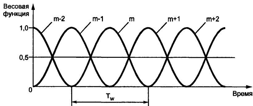
m-1, m, m+1 — последовательность измерительных окон, T_w — ширина измерительного окна
