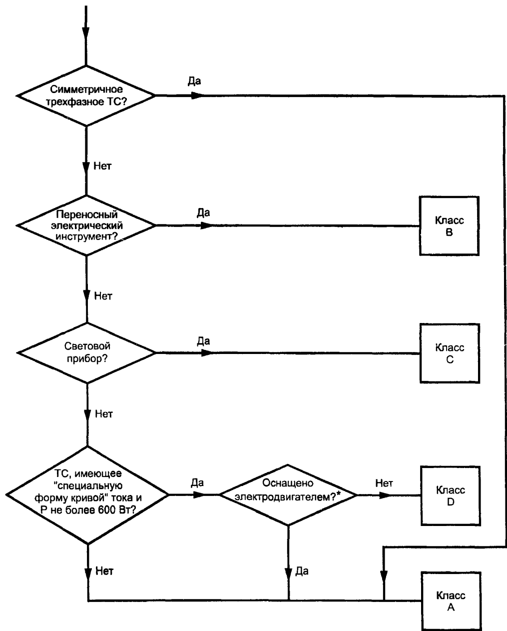
Рисунок 2 — Алгоритм классификации ТС
