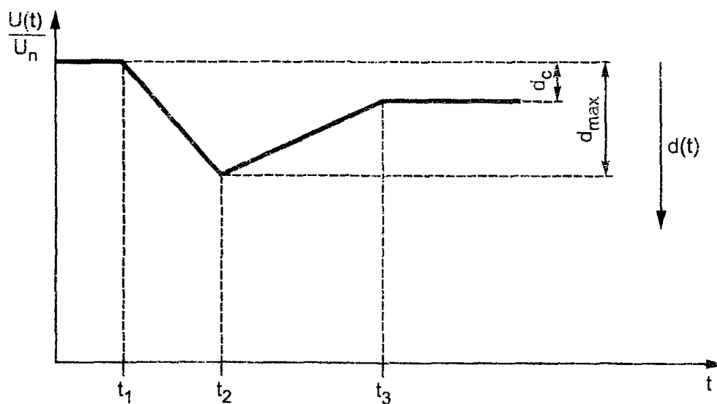
Рисунок 3 — Характеристика относительного изменения напряжения
