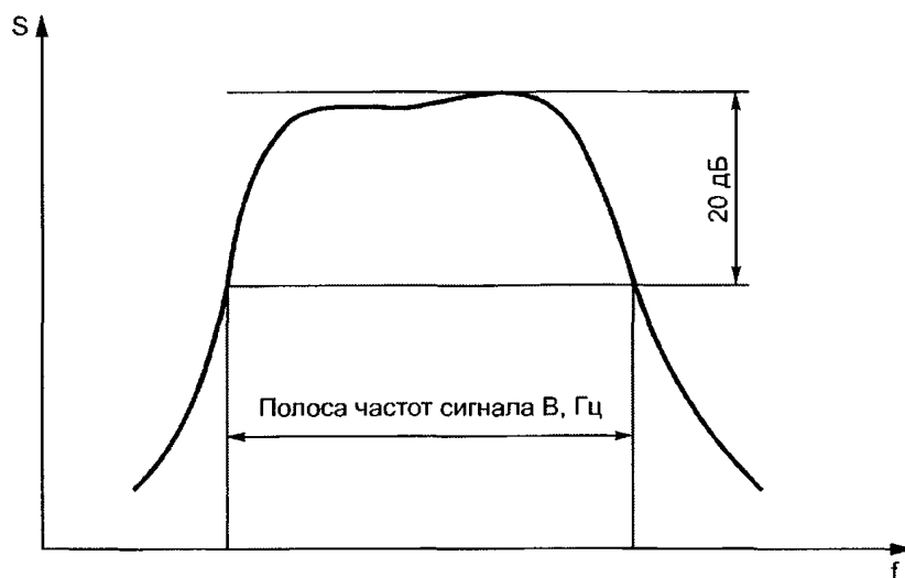
Рисунок 3 — Измерение полосы частот сигнала
