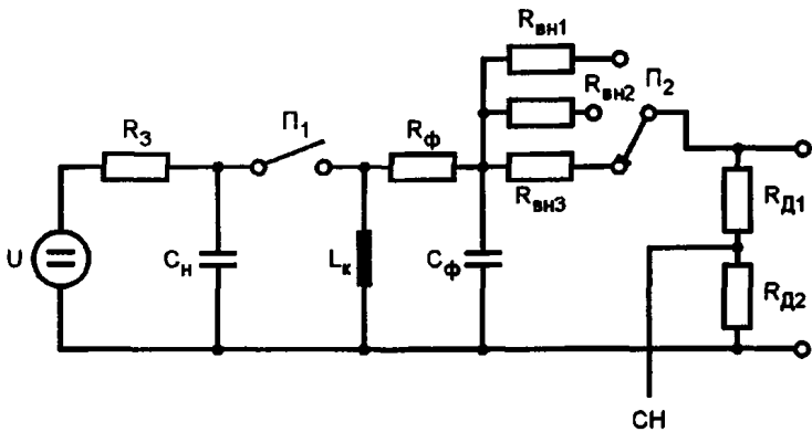
U — источник высокого напряжения; R — зарядный резистор; C_n — накопительный конденсатор; \Pi_1 — высоковольтный ключ; L_k — индуктивность колебательного контура; R_\phi — резистор фильтра; C_\phi — конденсатор фильтра; R_{н1} — резистор 12 Ом; R_{н2} — резистор 30 Ом; R_{н3} — резистор 200 Ом; \Pi_2 — селектор выходного сопротивления; R_{д1} , R_{д2} — резисторы делителя напряжения; CH — сигнал для наблюдения
