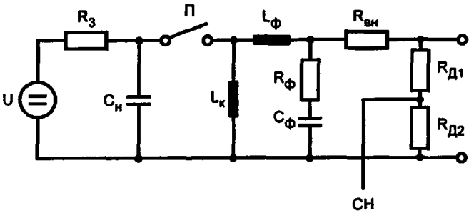
U — источник высокого напряжения; R_3 — зарядный резистор; C_n — накопительный конденсатор; \Pi — высоковольтный ключ; L_k — индуктивность колебательного контура; L_\phi — индуктивность фильтра; R_\phi — резистор фильтра; C_\phi — конденсатор фильтра; R_{н1} — резистор выходного сопротивления; R_{д1} , R_{д2} — резисторы делителя напряжения; CH — сигнал для наблюдения
