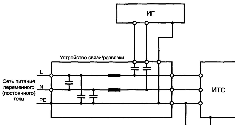
Рисунок 116 — Схема рабочего места с проводниками заземления (см. 7.1.2)
