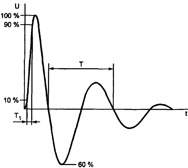
T_1 — время нарастания (0,5 мкс для напряжения в режиме холостого хода, 1 мкс для тока в режиме короткого замыкания); T — период колебаний (10 мкс) Рисунок 1 — Типовая форма одиночной КЗП (напряжение в режиме холостого хода и ток в режиме короткого замыкания)
