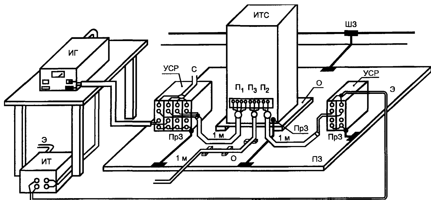
ШЗ — шина защитного заземления; Э — к сети электропитания; P_1 — порт ввода-вывода; P_2 — порт электропитания; P_3 — порт связи; С — к источнику сигналов; ПрЗ — проводник заземления; ПЗ — пластина заземления; УСР — устройство связи/развязки; О — изоляционная опора; ИТ — изолирующий трансформатор
