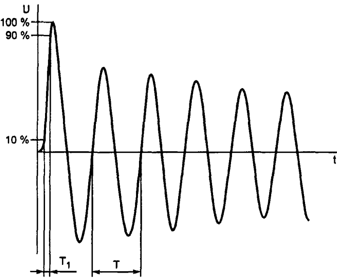
T_1 — время нарастания напряжения (75 нс); T — период колебаний (10 мкс для частоты 0,1 МГц, 1 мкс для частоты 1 МГц)
