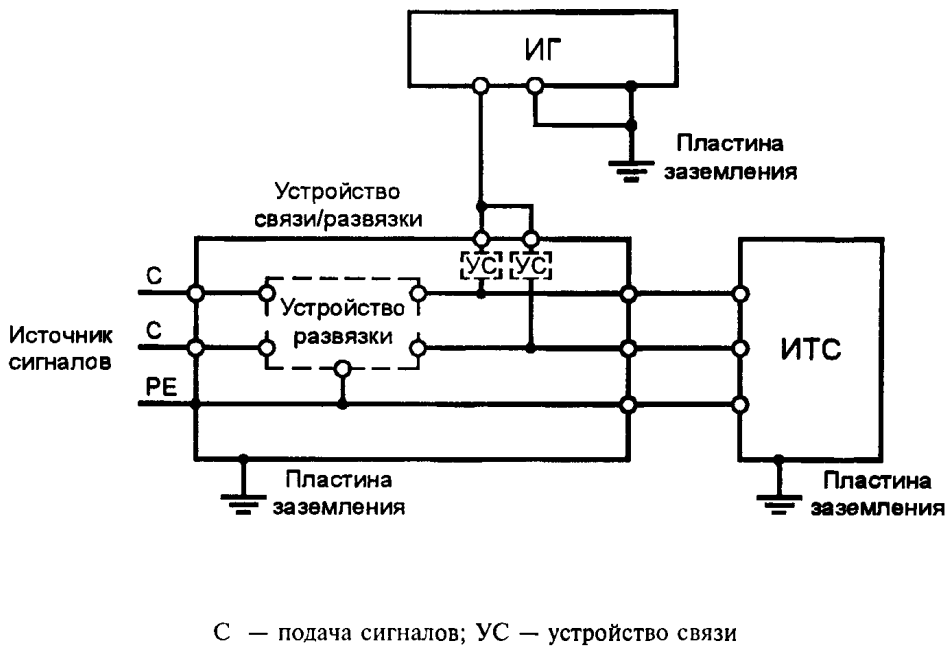
Рисунок 9а — Схема рабочего места с пластиной заземления (см. 7.1.1)
