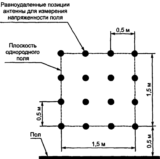
Рисунок 3 — Расположение оборудования при аттестации
