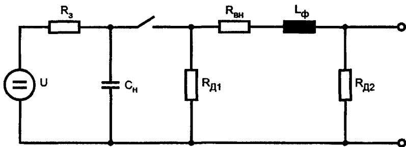
U — источник высокого напряжения; R 3 — зарядный резистор; C н — зарядный конденсатор; R д1 , R д2 — резисторы, определяющие длительность импульса; R вн — резистор, определяющий выходное полное сопротивление ИГ; L ф — индуктивность, определяющая время нарастания импульса
