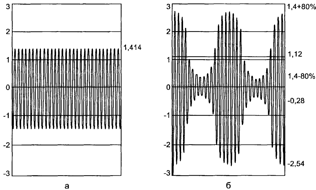
а — немодулированный радиочастотный сигнал (амплитудное значение напряжения U_i = 1,41 В; среднеквадратическое значение напряжения U_{\text{ср}} = 1 В); б — модулированный радиочастотный сигнал при глубине модуляции 80 % ( U_{\text{ср}} = 1,12 В; пиковое значение напряжения U_{\text{пик}} = 2,54 В)
