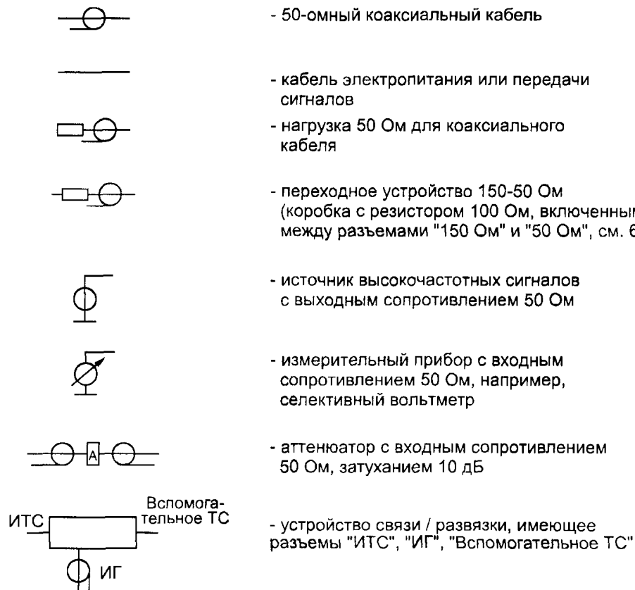
Рисунок 4а — Перечень символов, применяемых в приведенных ниже схемах рабочих мест для испытаний
