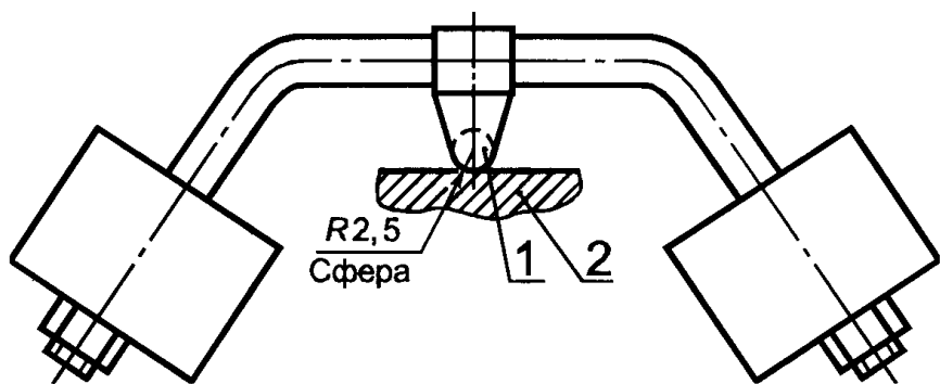
1 — стальной шарик; 2 — образец Рисунок 10 — Установка для испытаний давлением шарика
