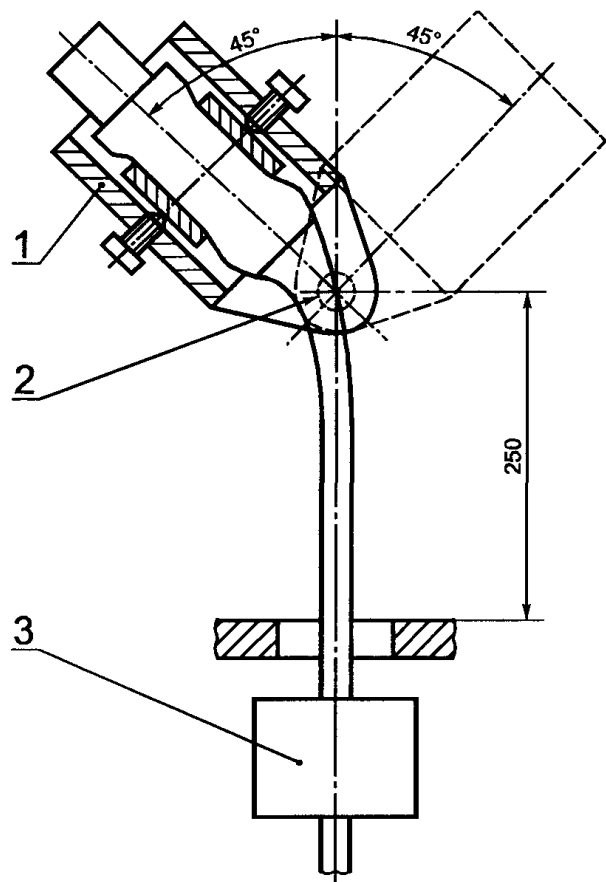
1 — устройство крепления образца; 2 — ось колебаний; 3 — груз Рисунок 9 — Устройство для испытания на изгиб
