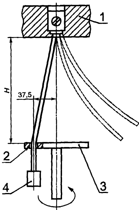
1 — панель; 2 — гильза; 3 — диск; 4 — груз Рисунок 15 — Установка для испытан- ний проводников на изгиб
