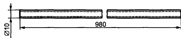
П р и м е ч а н и е — Материал детали — стальная труба с толщиной стенки 1 мм. Рисунок А.5 — Установка для испытаний на удар. Конструкция трубы
