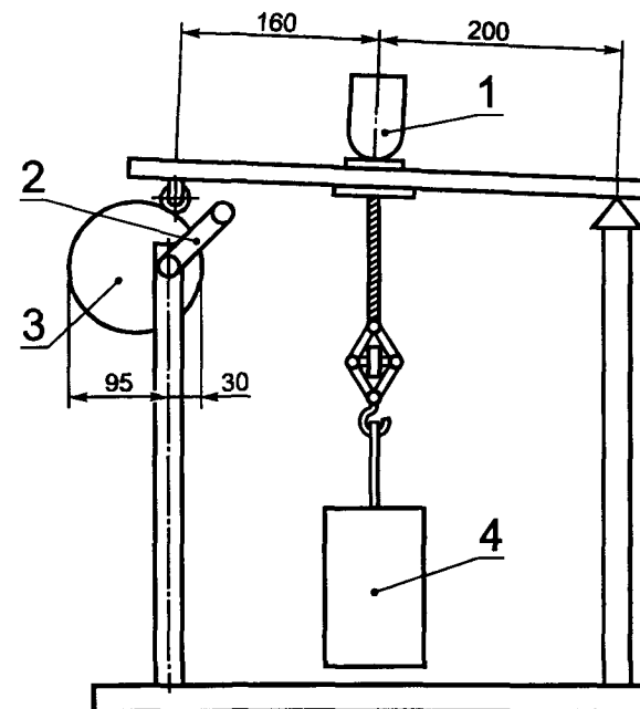
1 — испытуемый образец; 2 — колено; 3 — эксцентрик; 4 — груз
