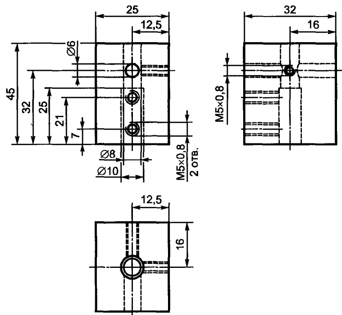
П р и м е ч а н и е — Материал детали — алюминий. Рисунок А.6 — Установка для испытаний на удар. Конструкция подвеса
