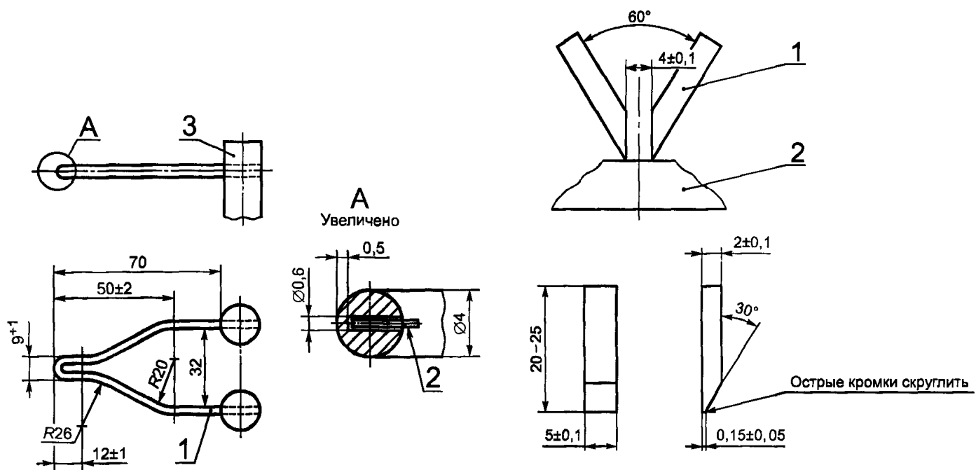
1 — раскаленная петля, запаянная в стойки; 2 — термопара; 3 — стойка
