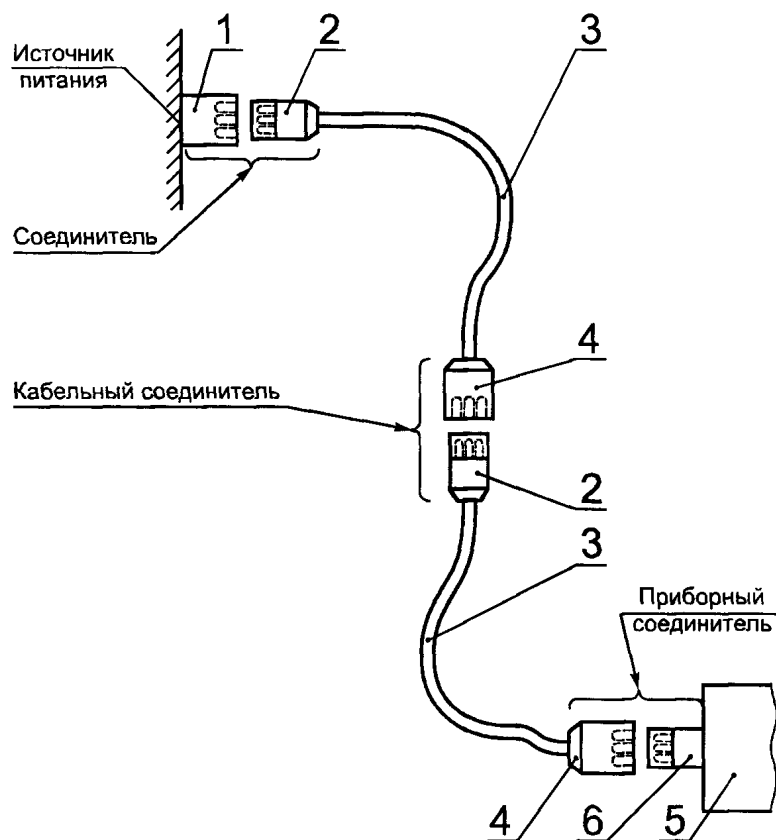
1 — панельная розетка; 2 — вилка; 3 — гибкий кабель; 4 — кабельная розетка; 5 — прибор; 6 — приборный ввод
