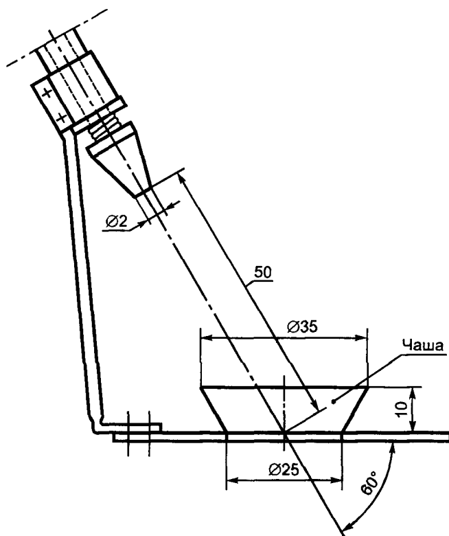
Рисунок 4 — Разбрызгиватель
