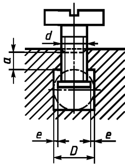
Зажим с прижимной пластиной
