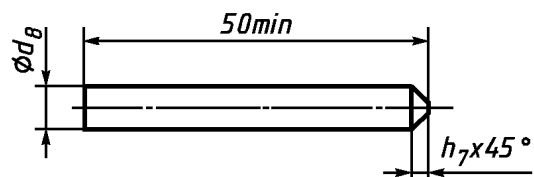
Рисунок 105 — Калибр для проверки фазных гнезд
