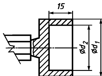
Калибр В для проверки диаметра d_2
