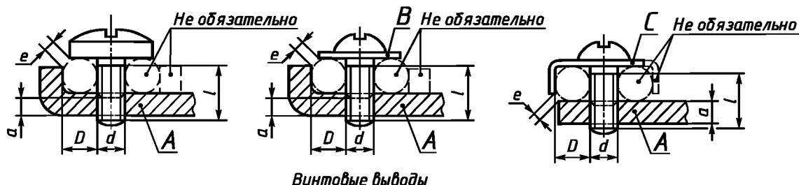
Винтовые выводы
