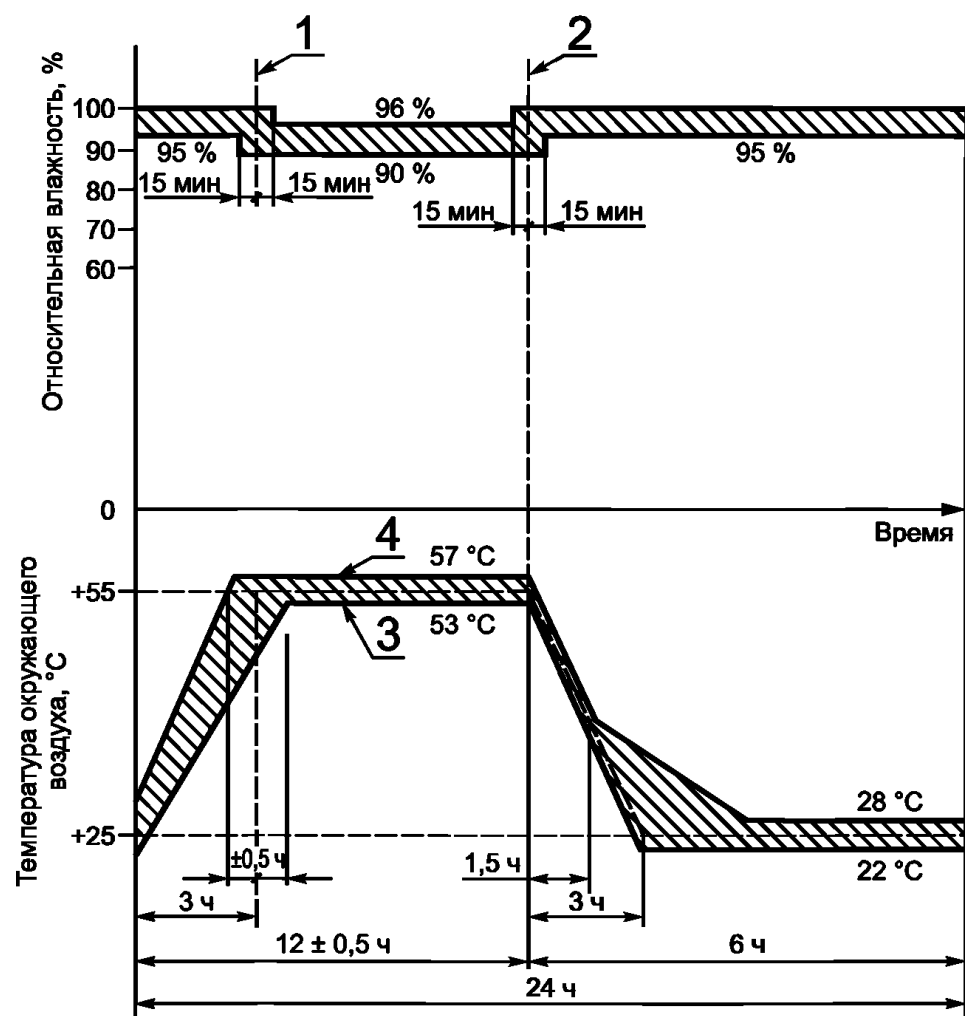
1 — конец повышения температуры; 2 — начало снижения температуры; 3 — нижнее значение температуры; 4 — верхнее значение температуры Рисунок 21 — Цикл испытаний на надежность (9.22.1.3)
