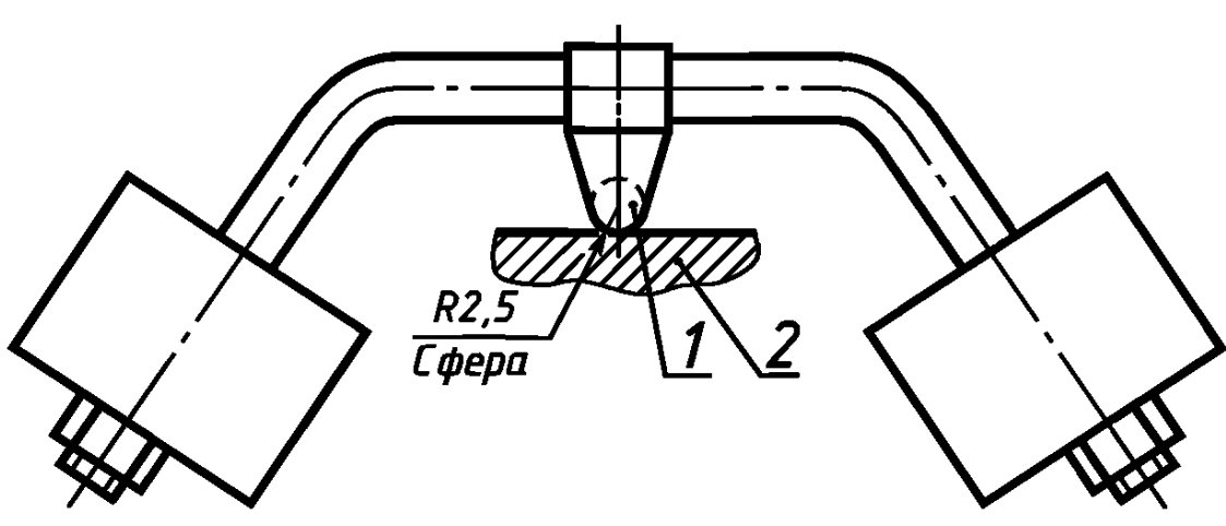
1 — стальной шарик диаметром 5 мм; 2 — образец Рисунок 18 — Аппарат для испытания давлением шарика (9.14.2)
