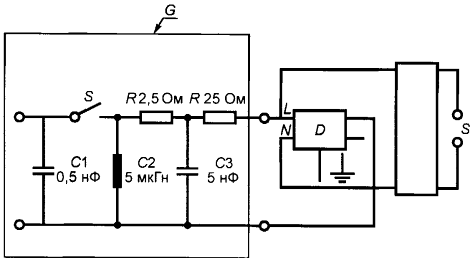
G — генератор затухания колебаний волны; D — АВДТ; S — источник питания; N — нулевой рабочий проводник; L — фазный проводник
