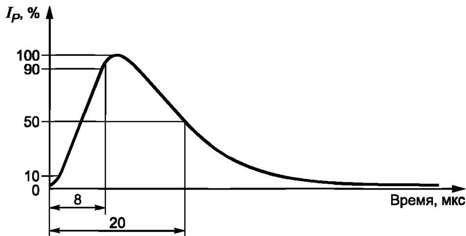
I_p — пиковый ток.
