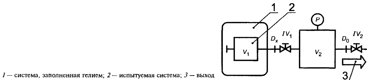
Рисунок Ж.1 — Схема испытания неповреждаемости
