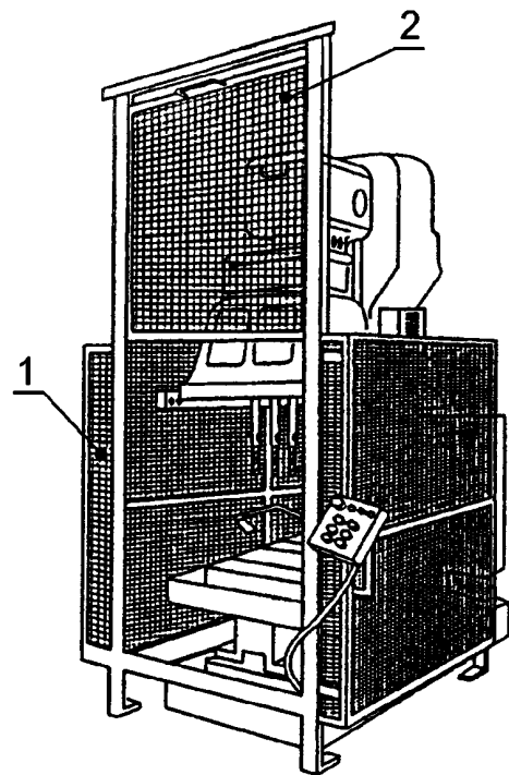
1 — съемное блокируемое устройство в открытом состоянии; 2 — съемное защитное устройство с фиксацией закрывания
