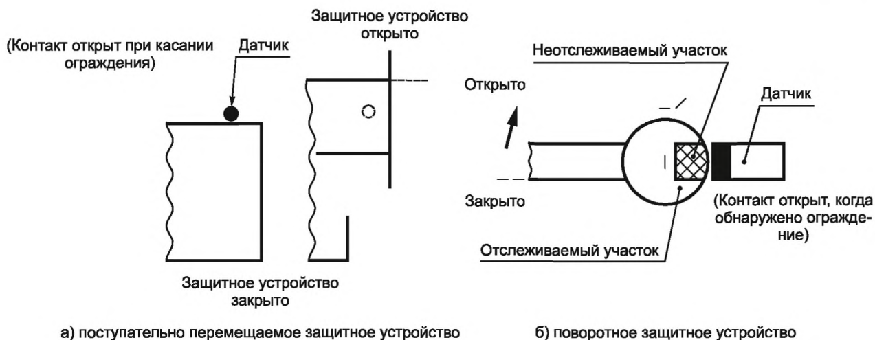
Рисунок 6 — Примеры защиты от вывода из строя бесконтактного переключателя
