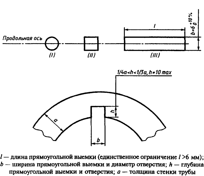
Рисунок 1 — Формы эталонных отверстия и выемок
