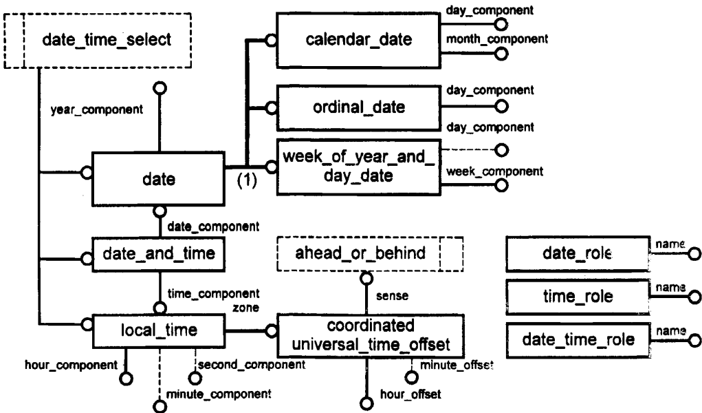
Рисунок F.13 — date_time_schema — EXPRESS-G диаграмма 1 из 1
