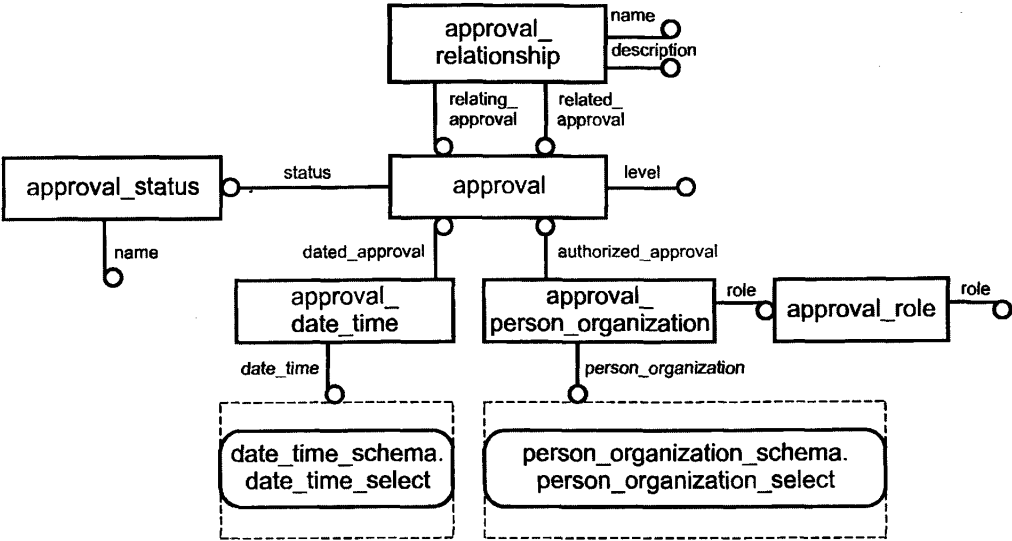
Рисунок F.9 — approval_schema — EXPRESS-G диаграмма 1 из 1
