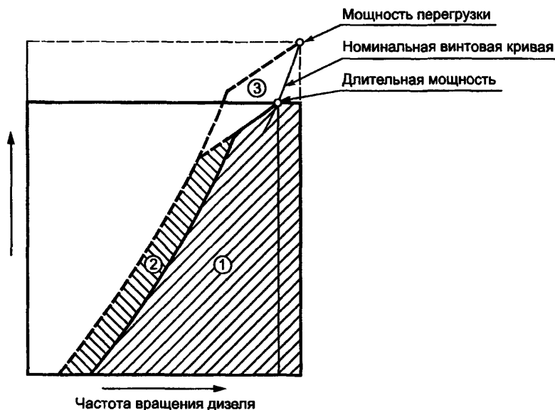
Рисунок 2 — Диаграмма «мощность — частота вращения»
