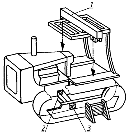
1 — балка для вертикального нагружения; 2 — заблокировано для предотвращения перемещения; 3 — блокировка противолесных трактов гусениц
