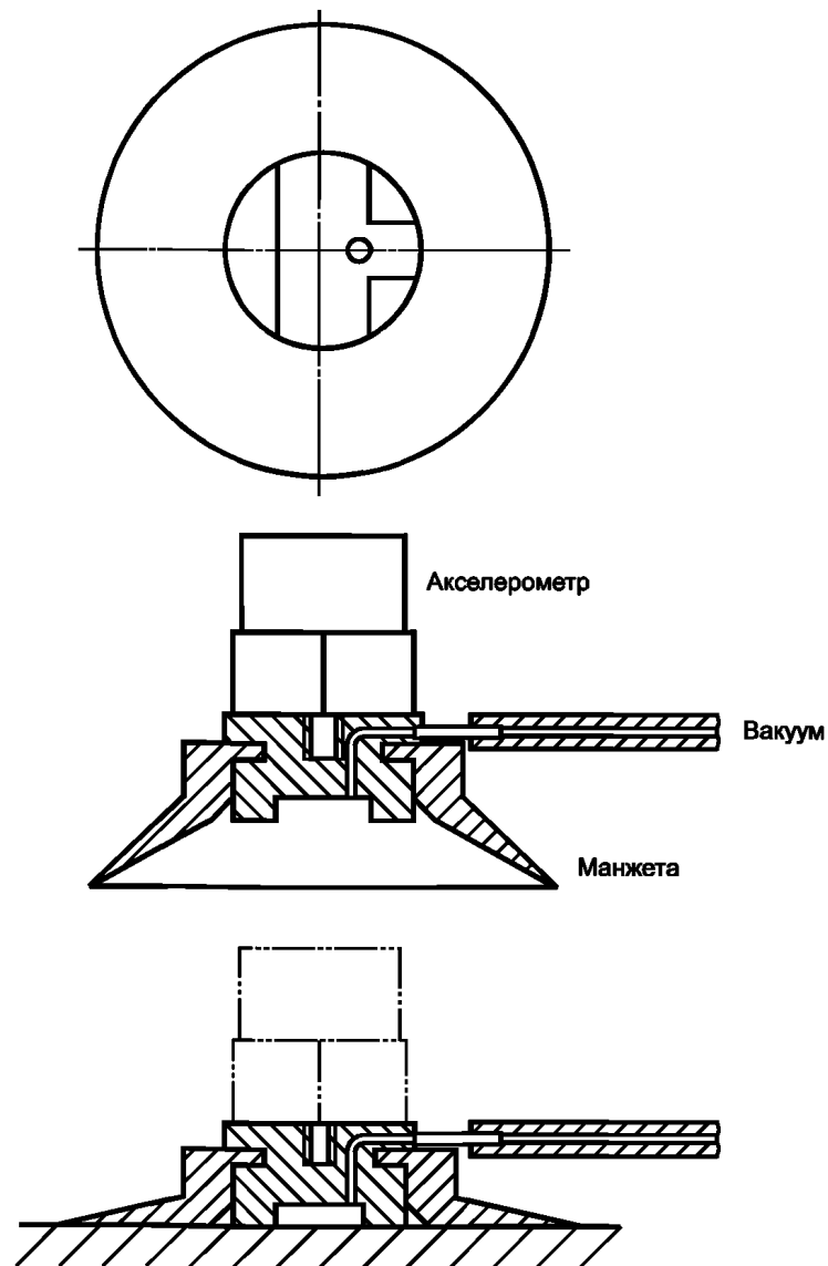
Рисунок 11 — Вакуумное крепление
