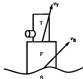
Рисунок 1 — Схематичное изображение установки акселерометра
