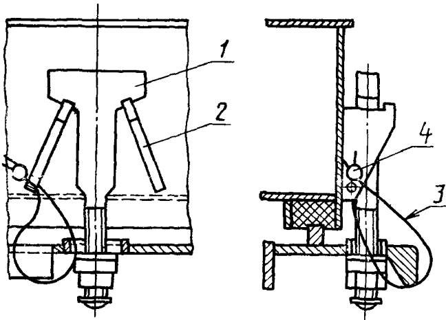
1 — задрайка, 2 — упор, 3 — связывающий элемент; 4 — пломба
