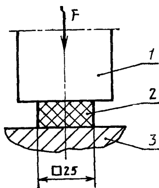
1 — силовой цилиндр (плунжер), 2 — образец типа 1; 3 — нагревательная плита
