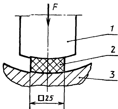
1 — силовой цилиндр (плунжер); 2 — образец типа 2, 3 — нагревательная плита
