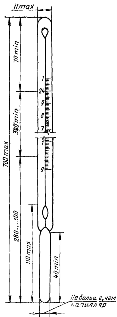
Рисунок 1 — Термометр палочный калориметри- ческий
