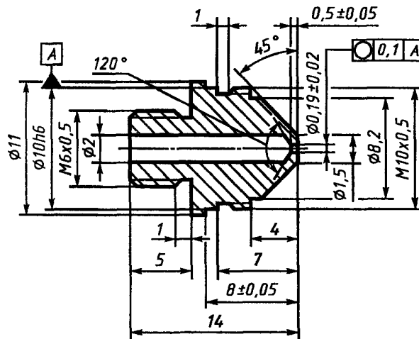
Рисунок Б.2 — Газовая форсунка
