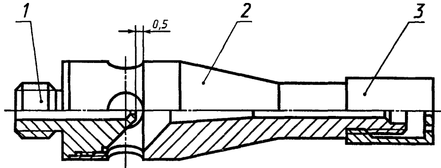
1 — газовая форсунка; 2 — трубка горелки; 3 — стабилизатор пламени
