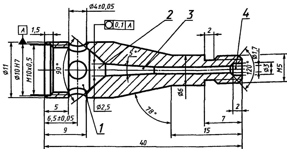
1 — воздушная камера; 2 — зона смешивания газа; 3 — зона рассеивания; 4 — выпускное отверстие
