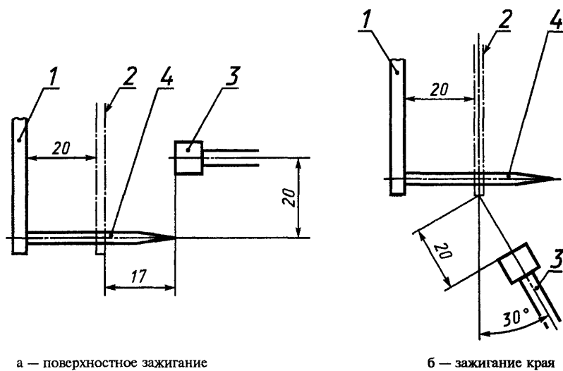
1 — рама держателя; 2 — элементарная проба; 3 — горелка; 4 — штифт
