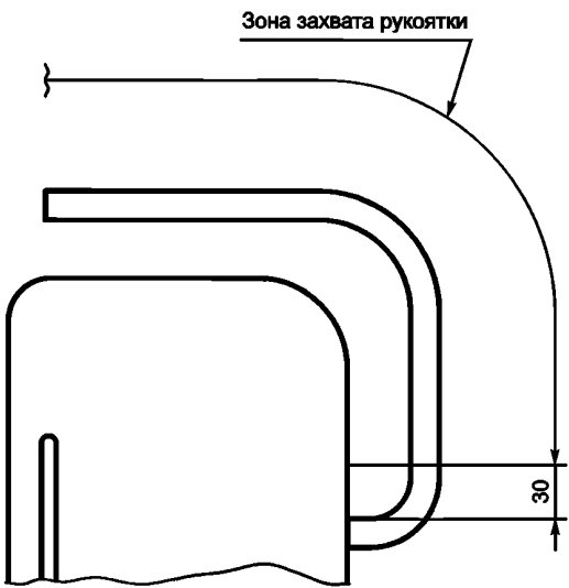
Рисунок 2 — Зона захвата рукоятки
