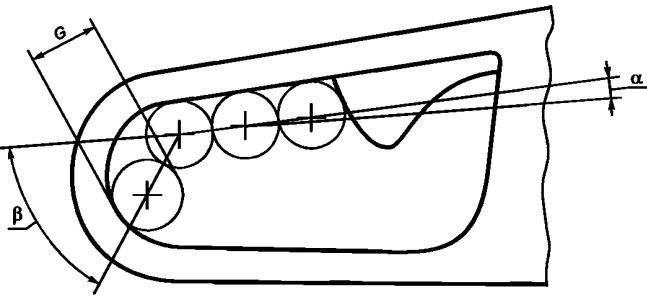
Рисунок 4 — Клиренсы за рычагом управления дросселем
