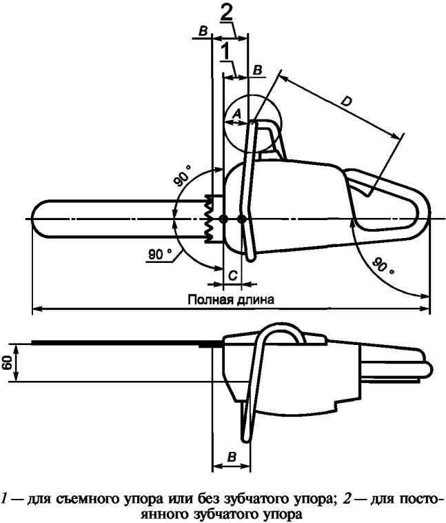
Рисунок 1 — Клиренсы передней рукоятки и расстояние между передней и задней рукоятками
