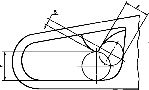
Рисунок 3 — Клиренсы у рычага управления дросселем
