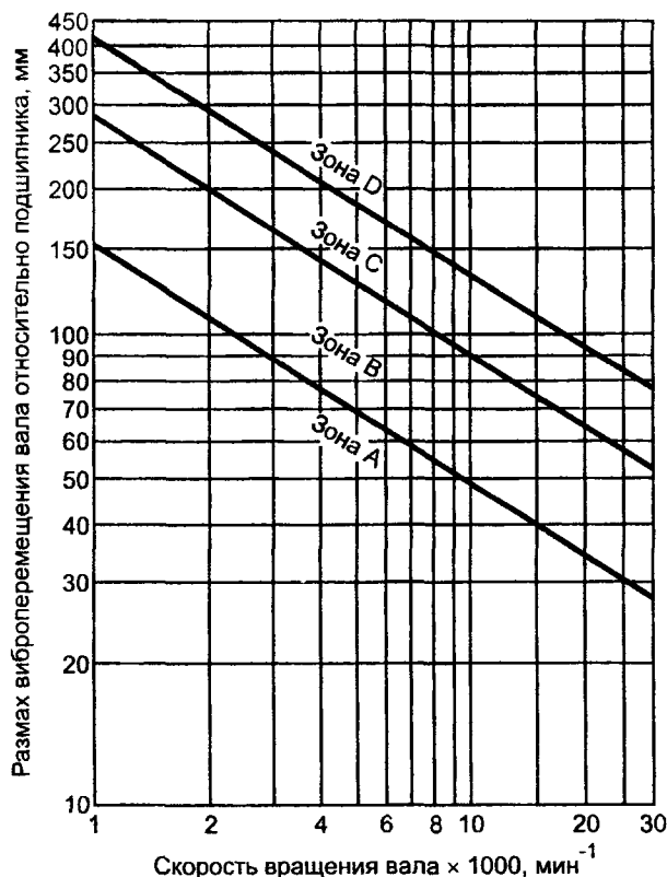
Рисунок А.1 — Рекомендуемые значения максимальных относительных перемещений вала в зависимости от максимальной рабочей скорости вращения вала машины
