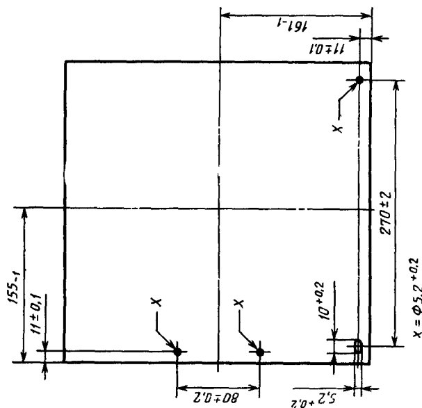
Форматная пленка S_4 297×297 мм. Размеры и расположение установочных отверстий и средней просеиваемой области
