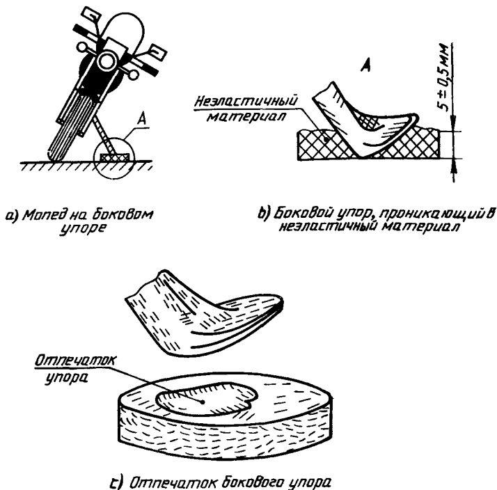
Рисунок 1 — Боковой упор
