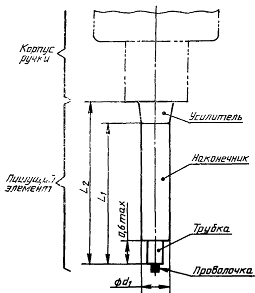
Рисунок 1 — Наконечник трубчатый
