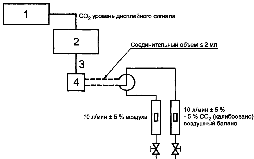
1 — самописец или осциллоскоп; 2 — капнометр; 3 — трубка образца; 4 — датчик или адаптер для трубки образца
